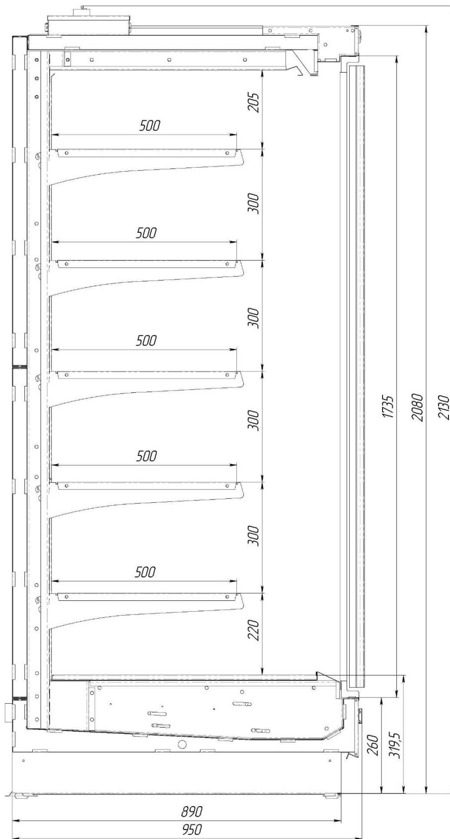
рисунок 2.1 – Сечение витрины VRIII2080.950 ESC
