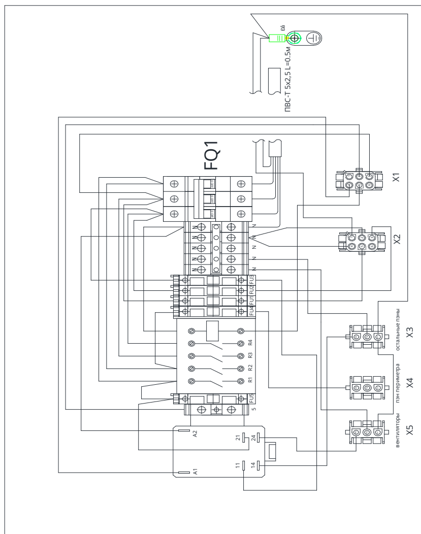
Схема электрическая монтажная блока электроники ODISSEY ST Горка 250/375 (CAREL)
