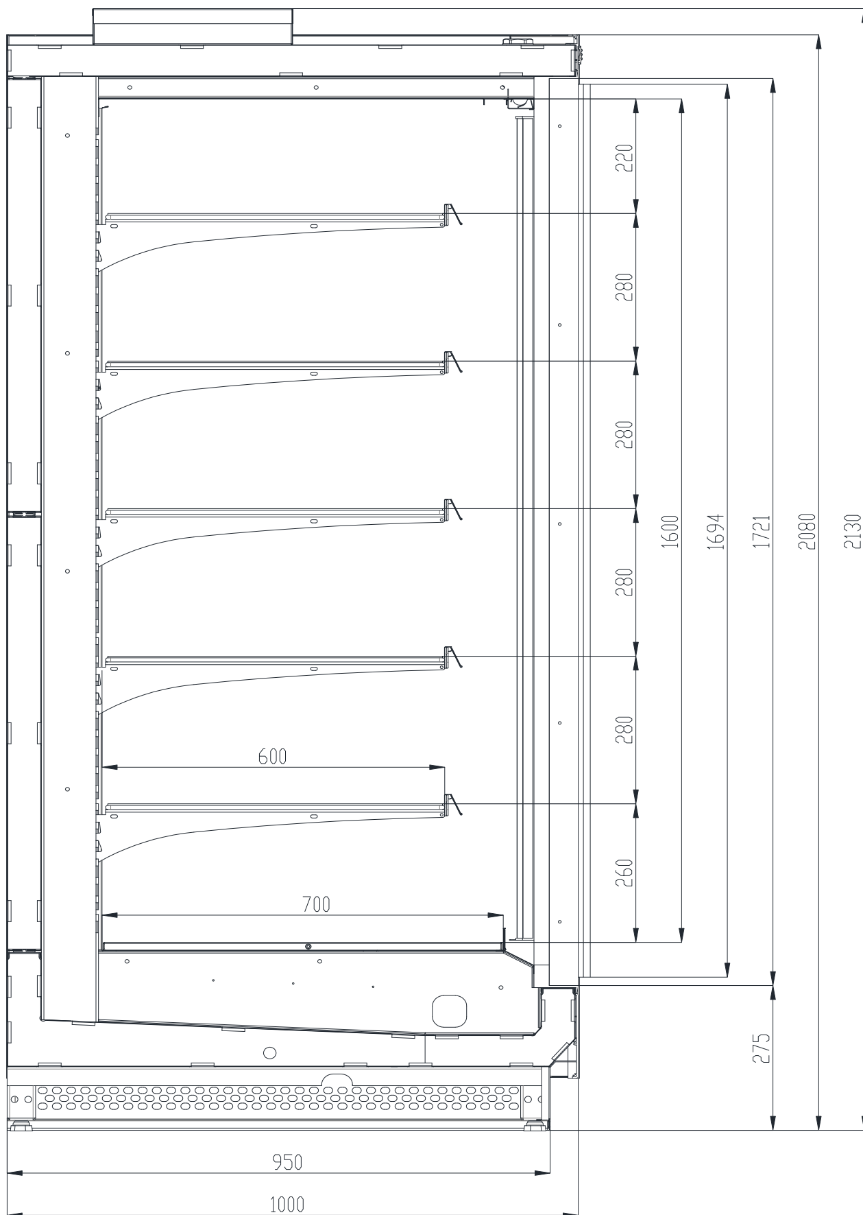
рисунок 2.1 – Сечение ODISSEY-II
