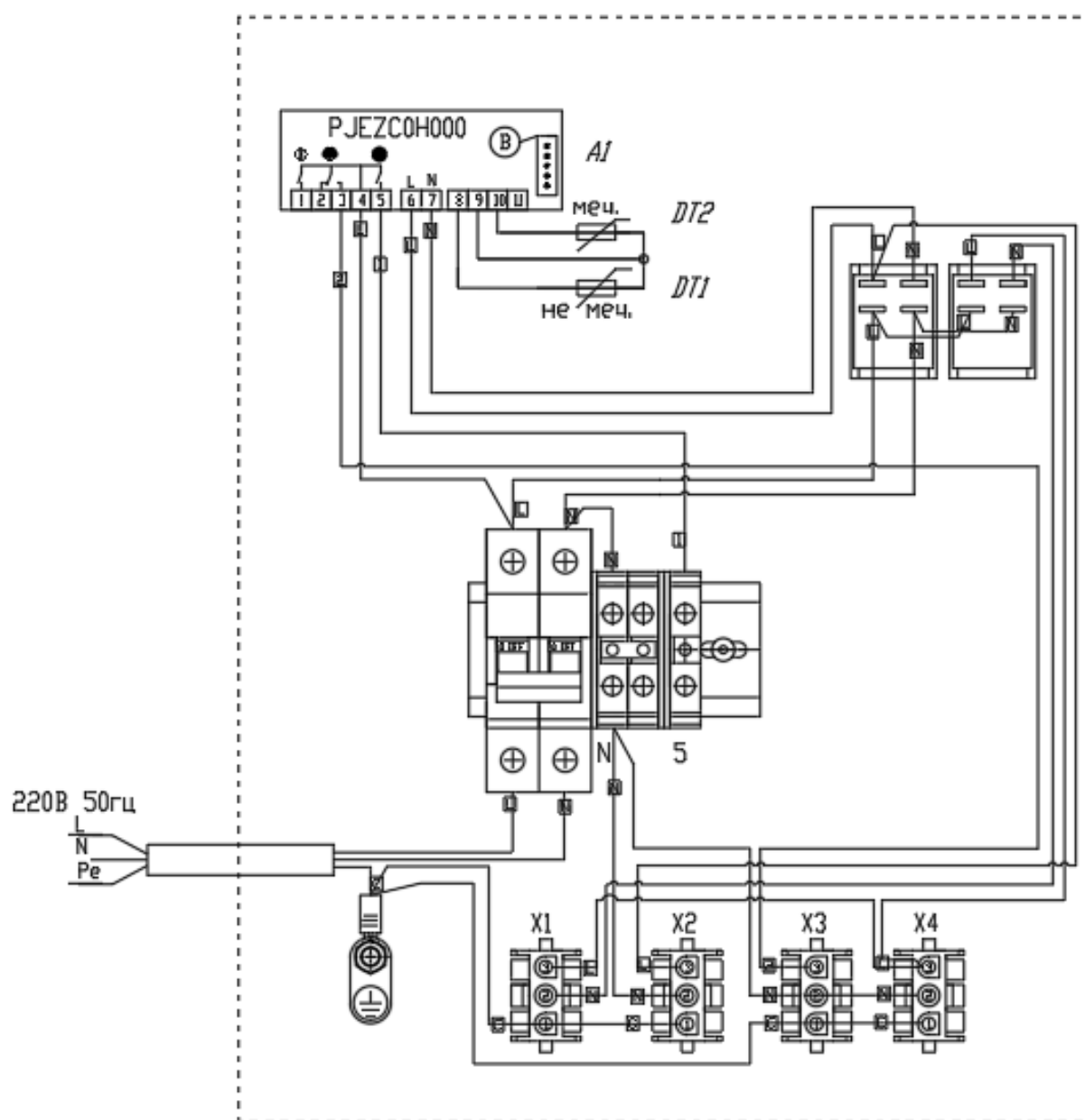
Схема электрическая монтажная блока электроники CAREL с выносным холодильным агрегатом
