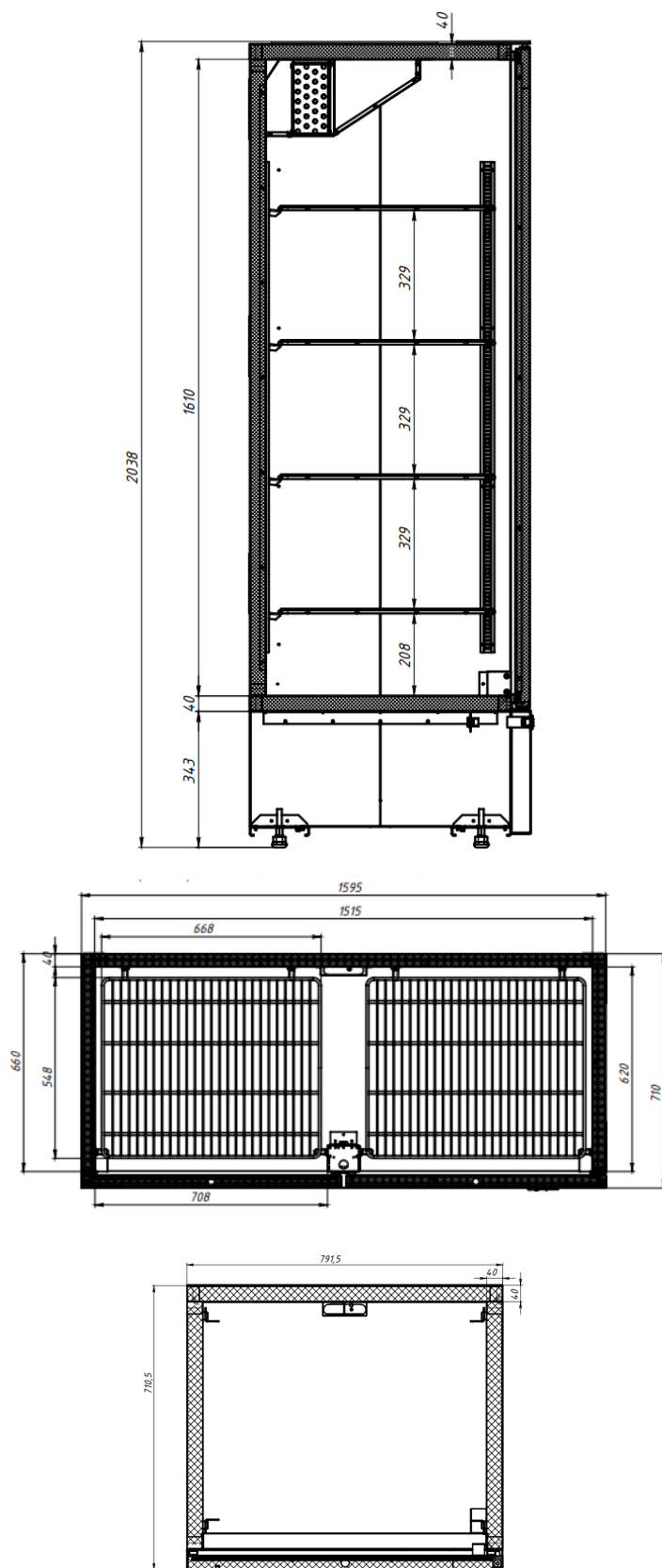
рисунок 2 – Сечение шкафа холодильного «Shkaff СТ 1400 и 700»
