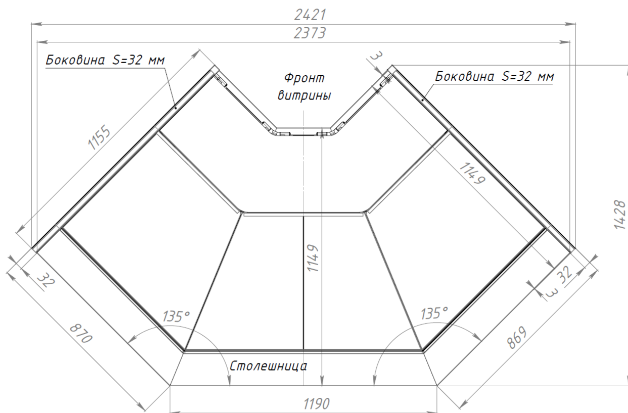
Витрина CALYPSO 3Y 90 (вид сверху)
