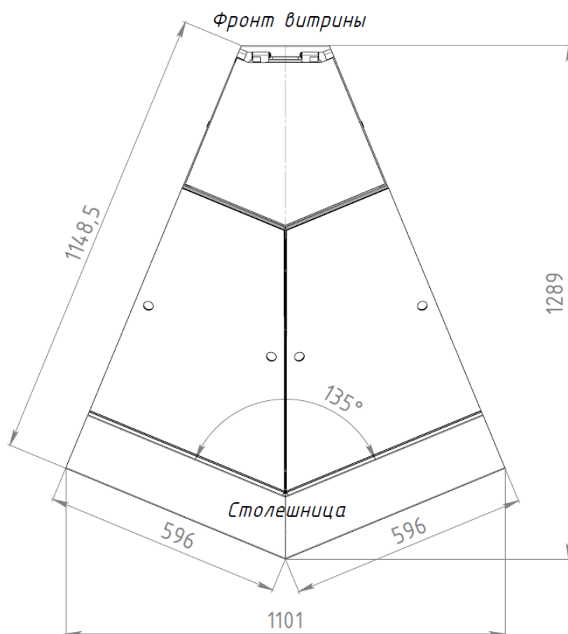
Витрина CALYPSO 3У 45 (вид сверху)
