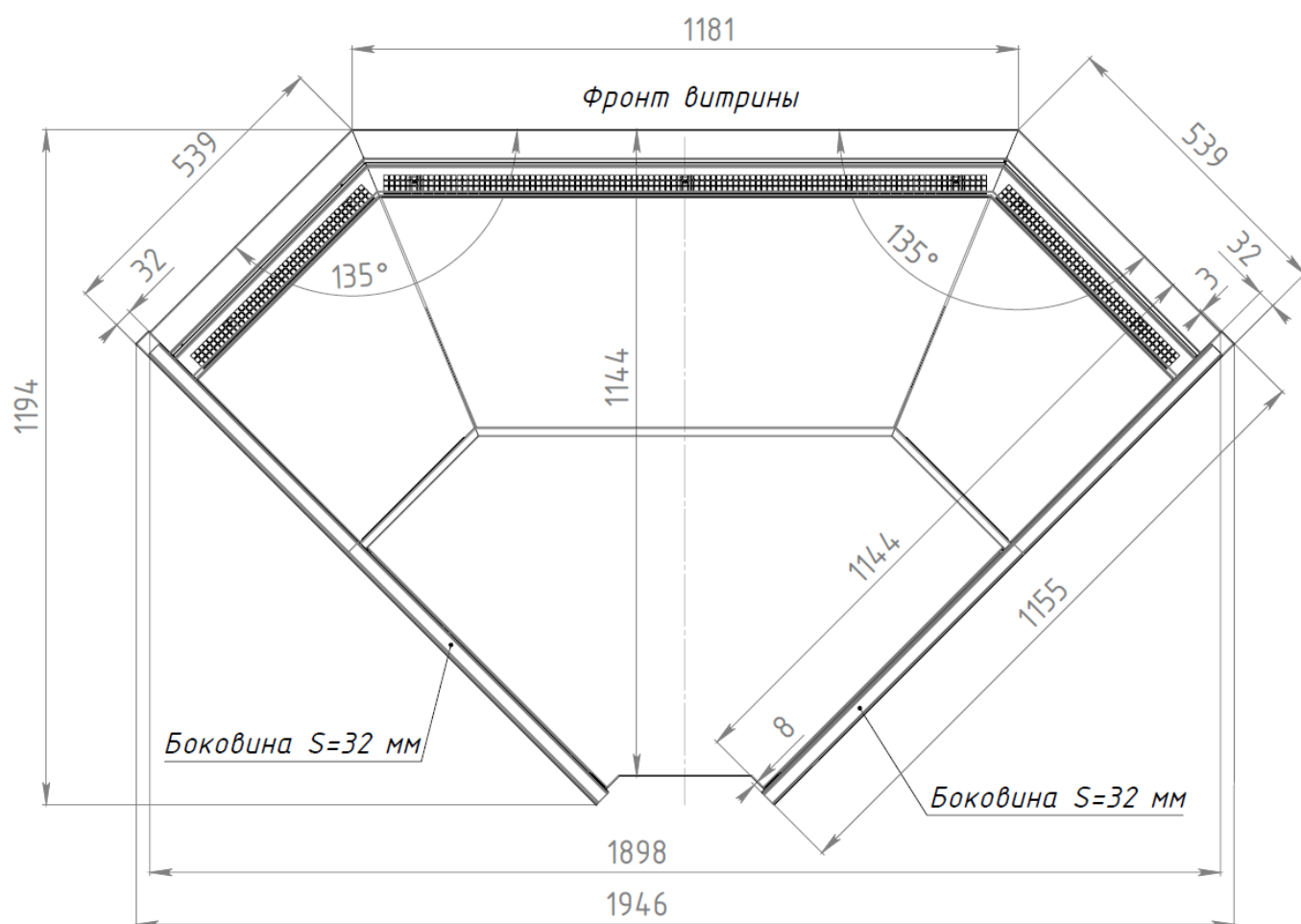
Витрина CALYPSO OY TOP LIGHT (вид сверху)
