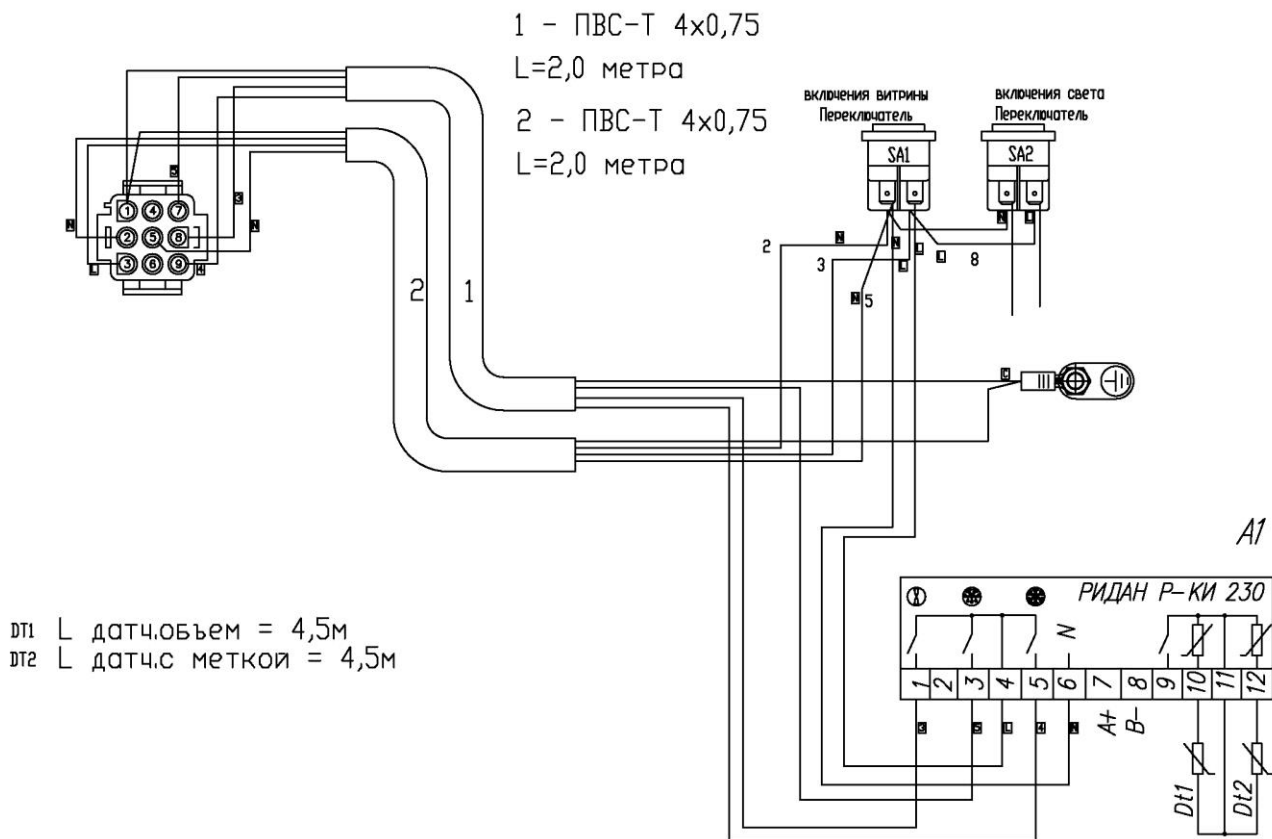
Схема электрическая монтажная кабельного шлейфа CRONOX PLUG-IN 250 РИДАН Р-КИ 230
