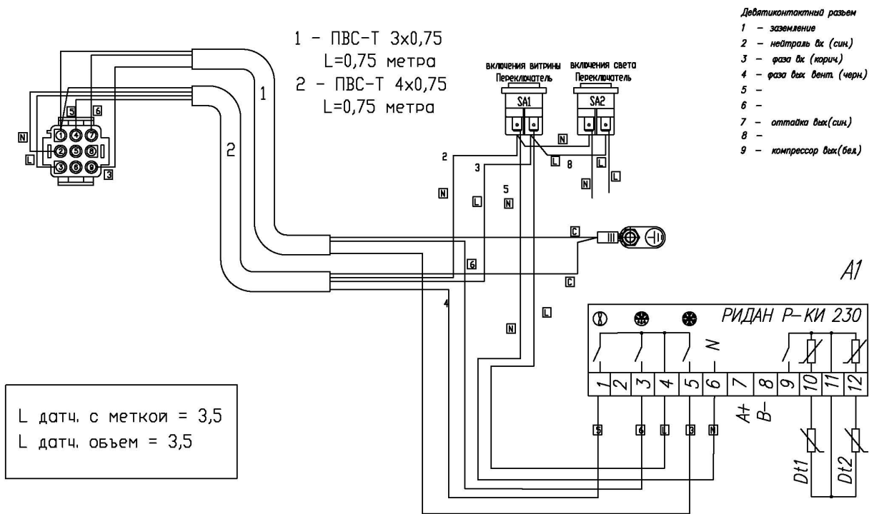
Схема электрическая монтажная кабельного шлейфа CRONOX plug in под РИДАН Р-КИ 230
