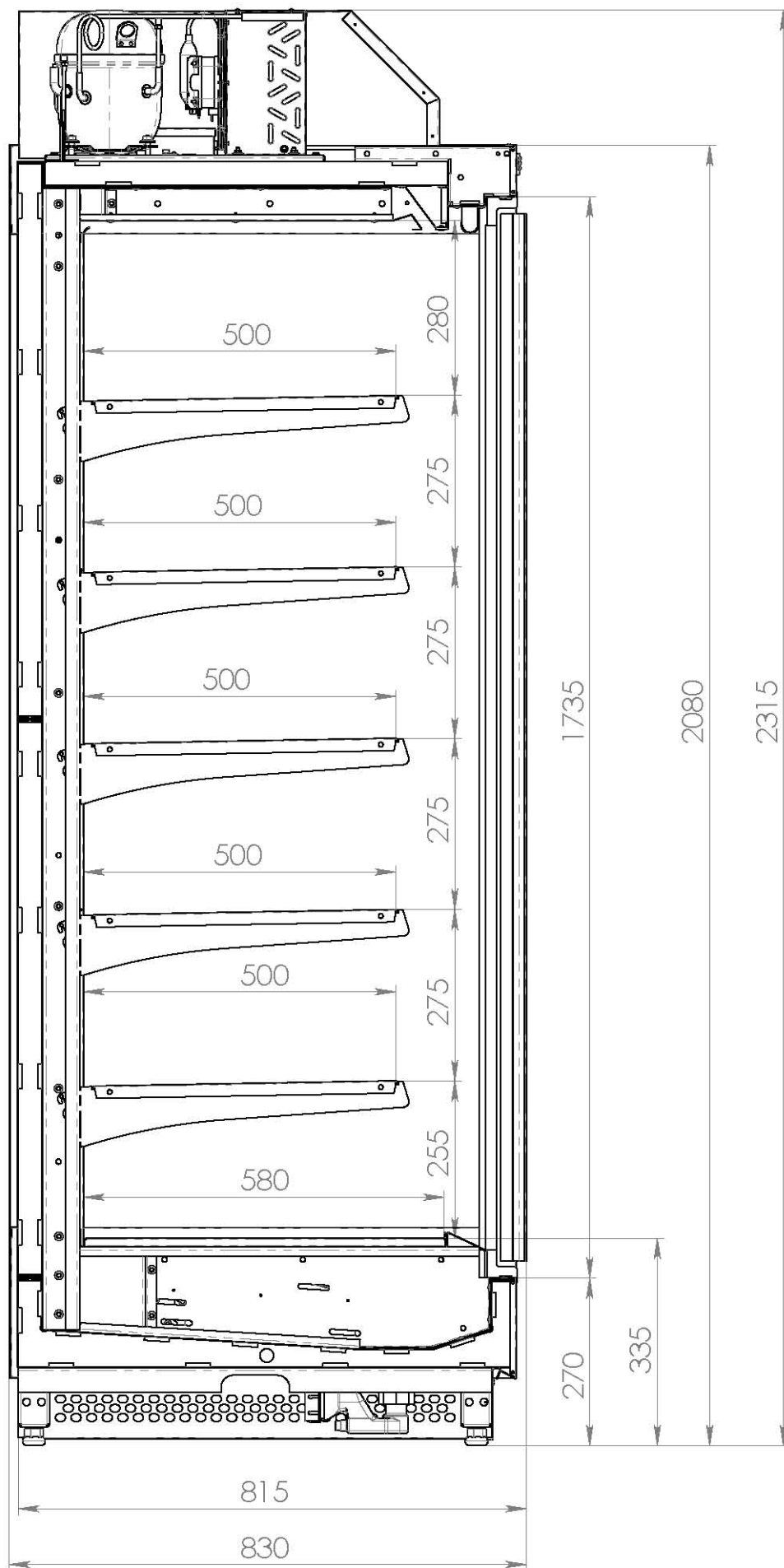
рисунк 2.2 – Сечение витрины CRONOX.2080.800 ESC
