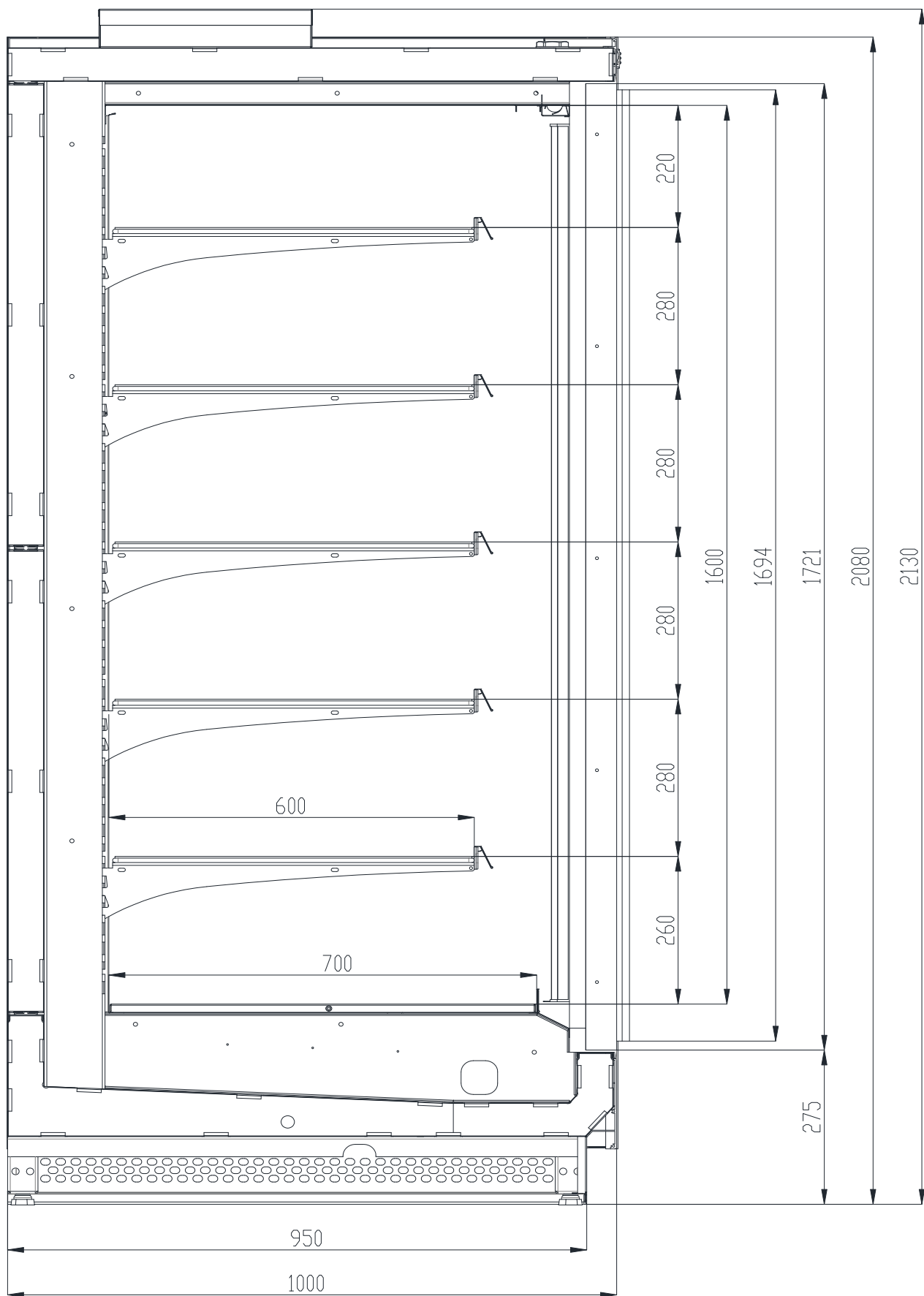
рисунок 2.1 – Сечение ODISSEY-II
