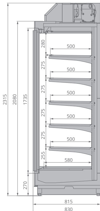
CRONOX.2080.800 ESC
