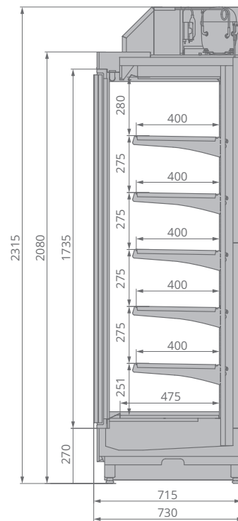
CRONOX.2080.700 ESC
