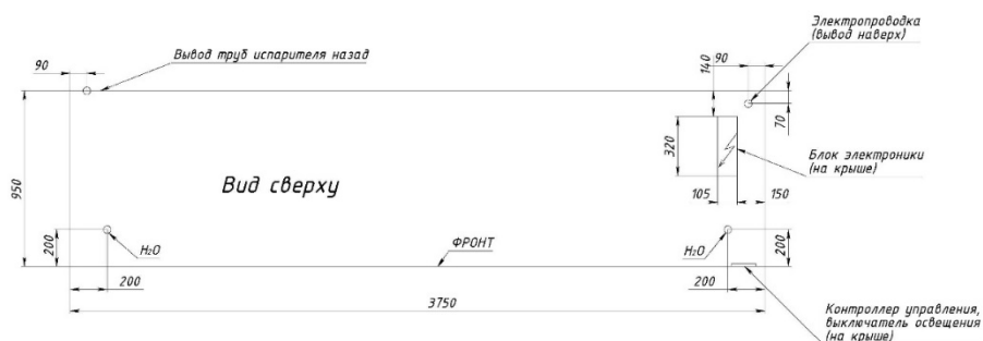
Схема расположения патрубков на витринах VRIII.2080.950.375/250/125
