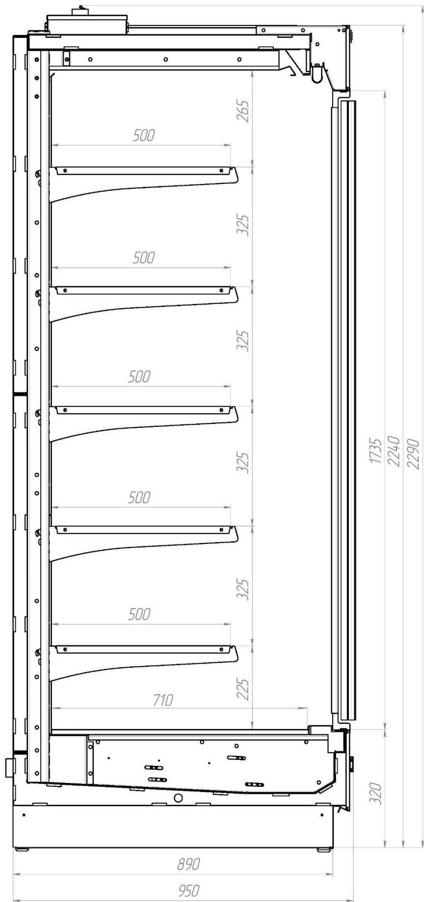
рисунок 2.1 – Сечение витрины VRIII2240.950 ESC
