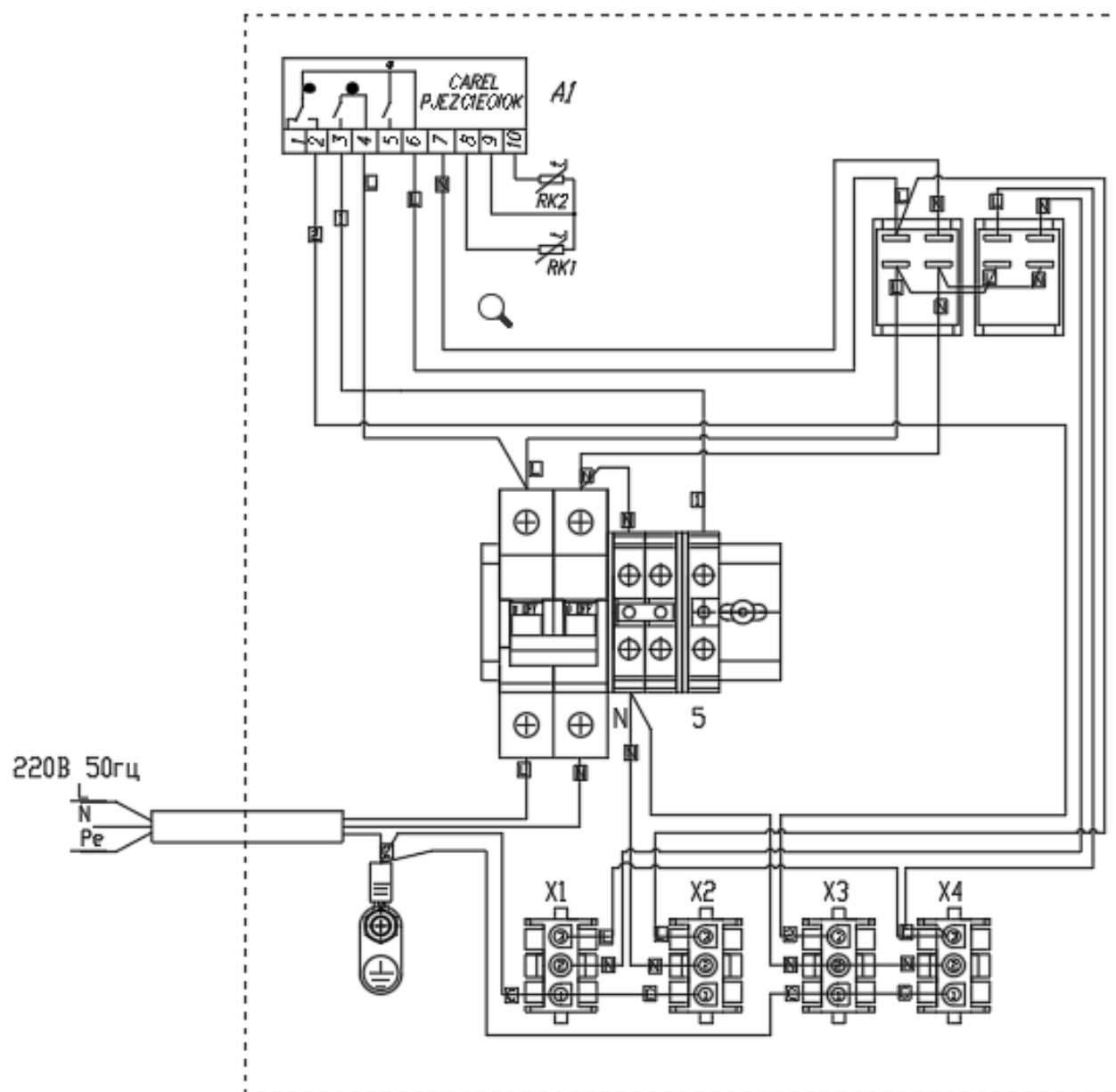
Схема электрическая монтажная блока электроники CAREL с выносным холодильным агрегатом
