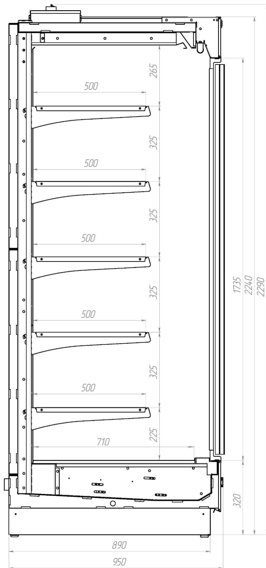
рисунок 2.1 – Сечение витрины VRIII2240.950 ESC
