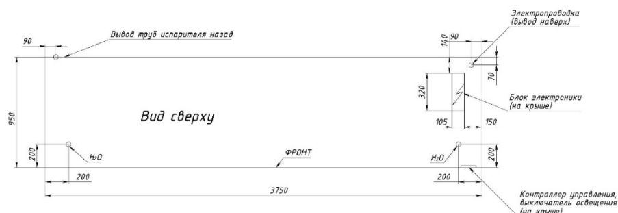
Схема расположения патрубков на витринах VRIII.2080.950.375/250/125
