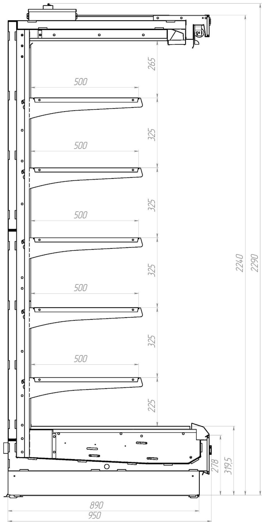
рисунок 2.2 – Сечение витрины VRIII2240.950
