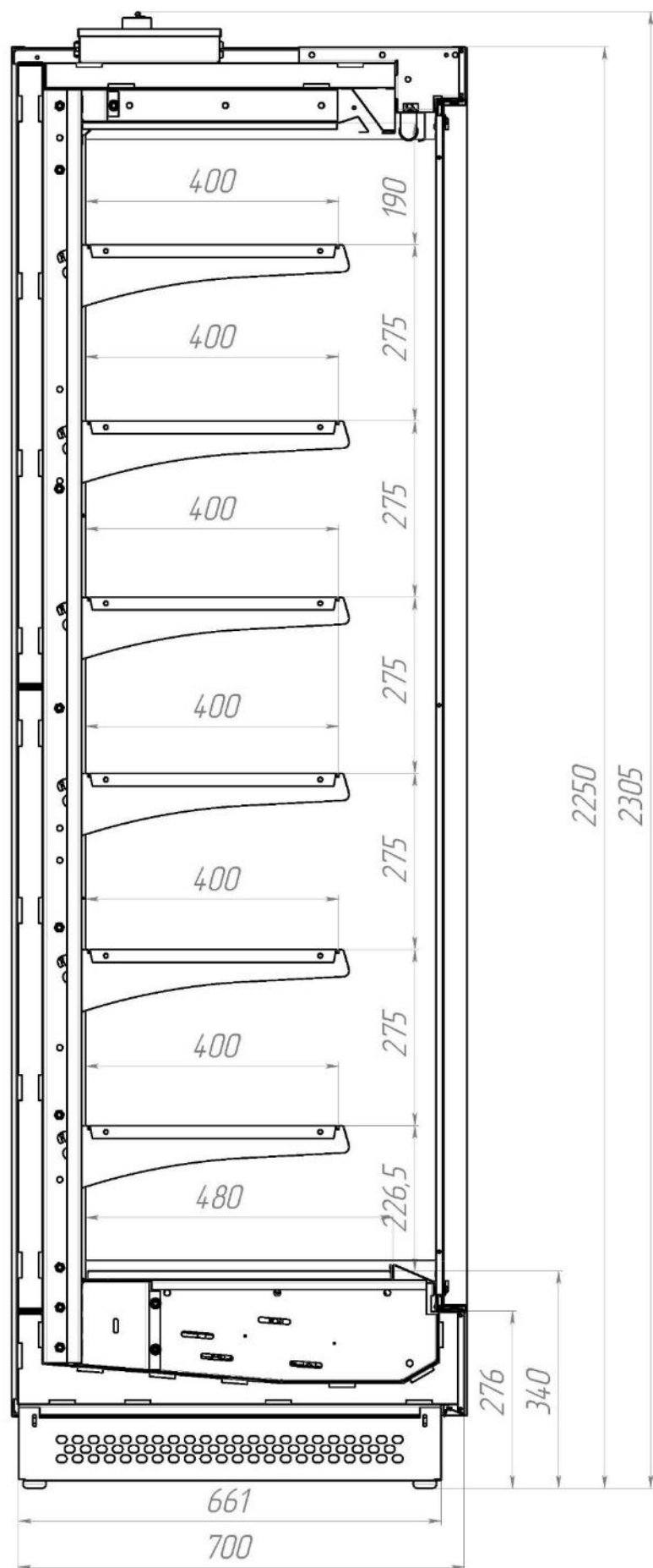
рисунок 2.4 – Сечение витрины TESEY III 2240 ULTRA SLIM
