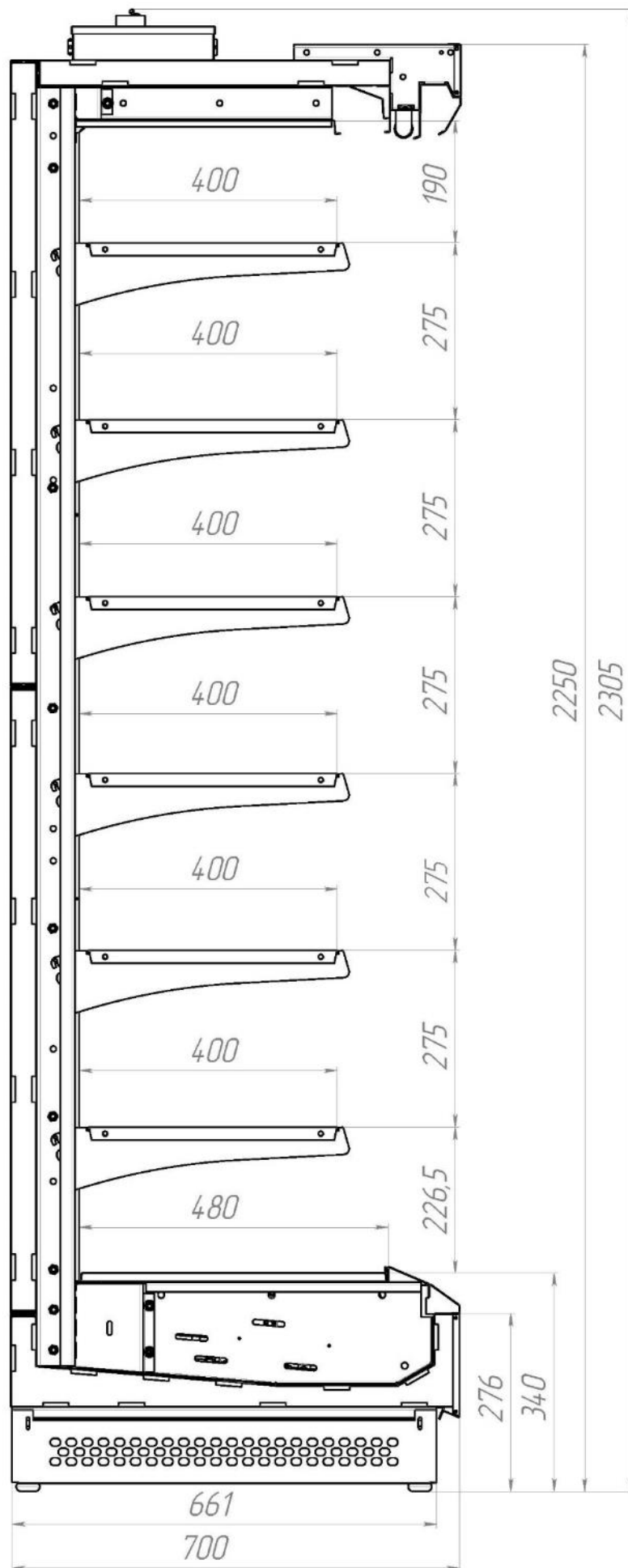
рисунок 2.3 – Сечение витрины TESEY III 2240 ULTRA SLIM
