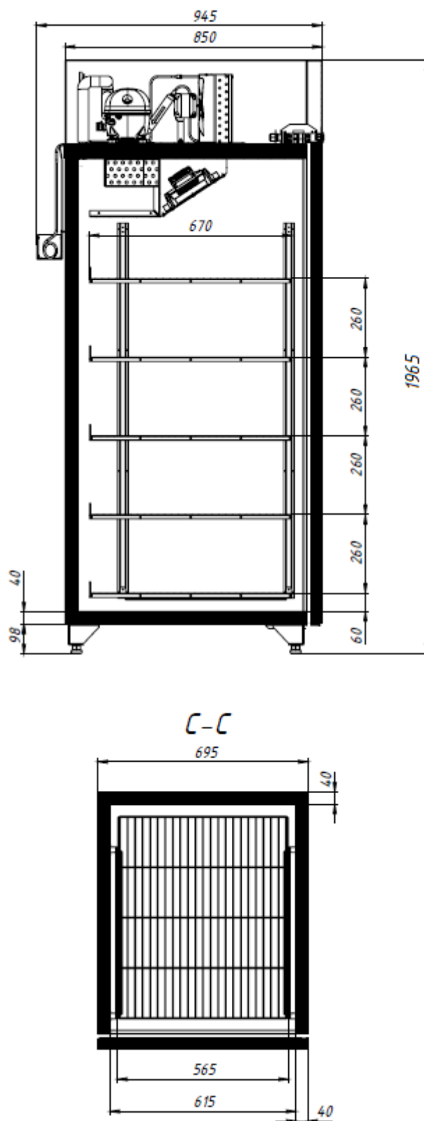
рисунок 5 – Сечение шкафа холодильного «Shkaff II 0,7 CT TOP»
