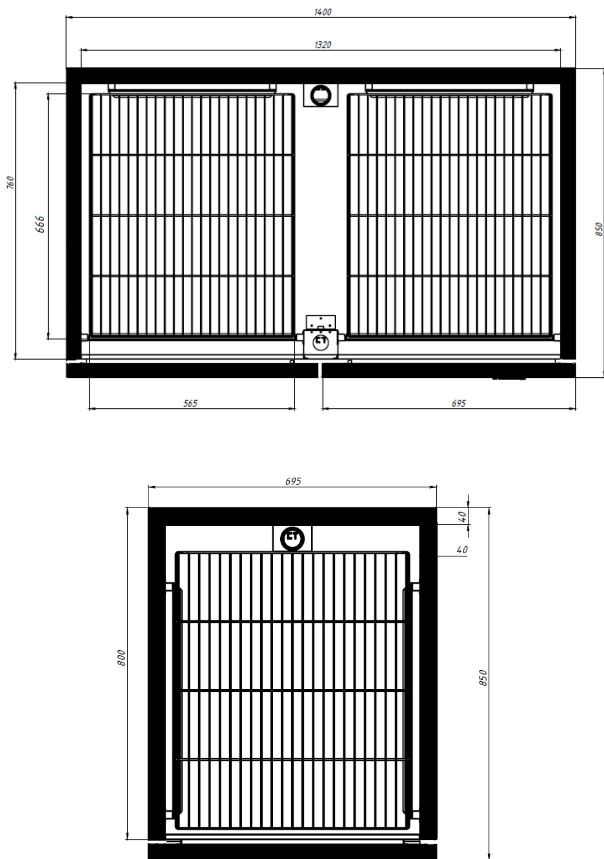
рисунок 3 – Сечение шкафа холодильного «Shkaff II 1400CT и 700CT»
