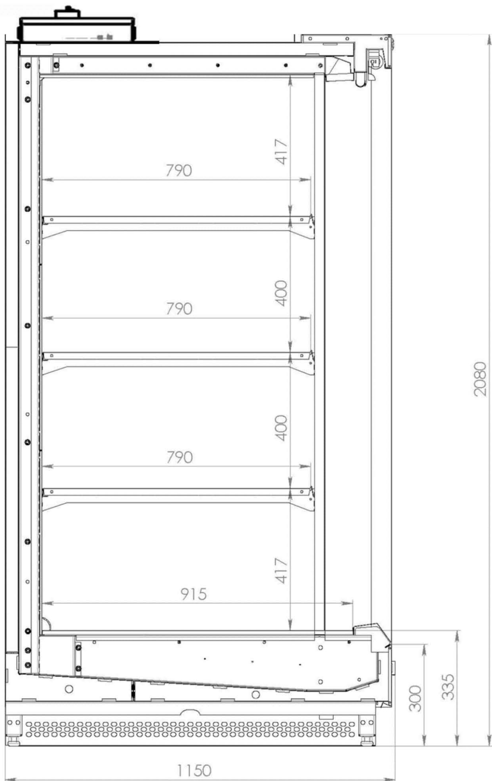
рисунок 2.8 – Сечение витрины VRIII2080.1200
