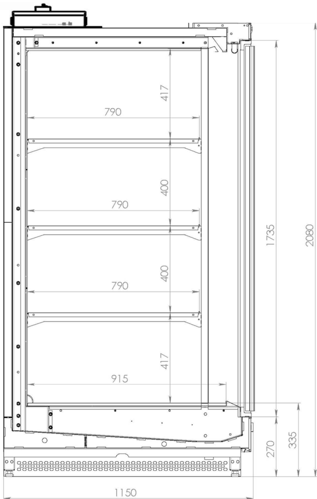
рисунок 2.7 – Сечение витрины VRIII2080.1200 ESC
