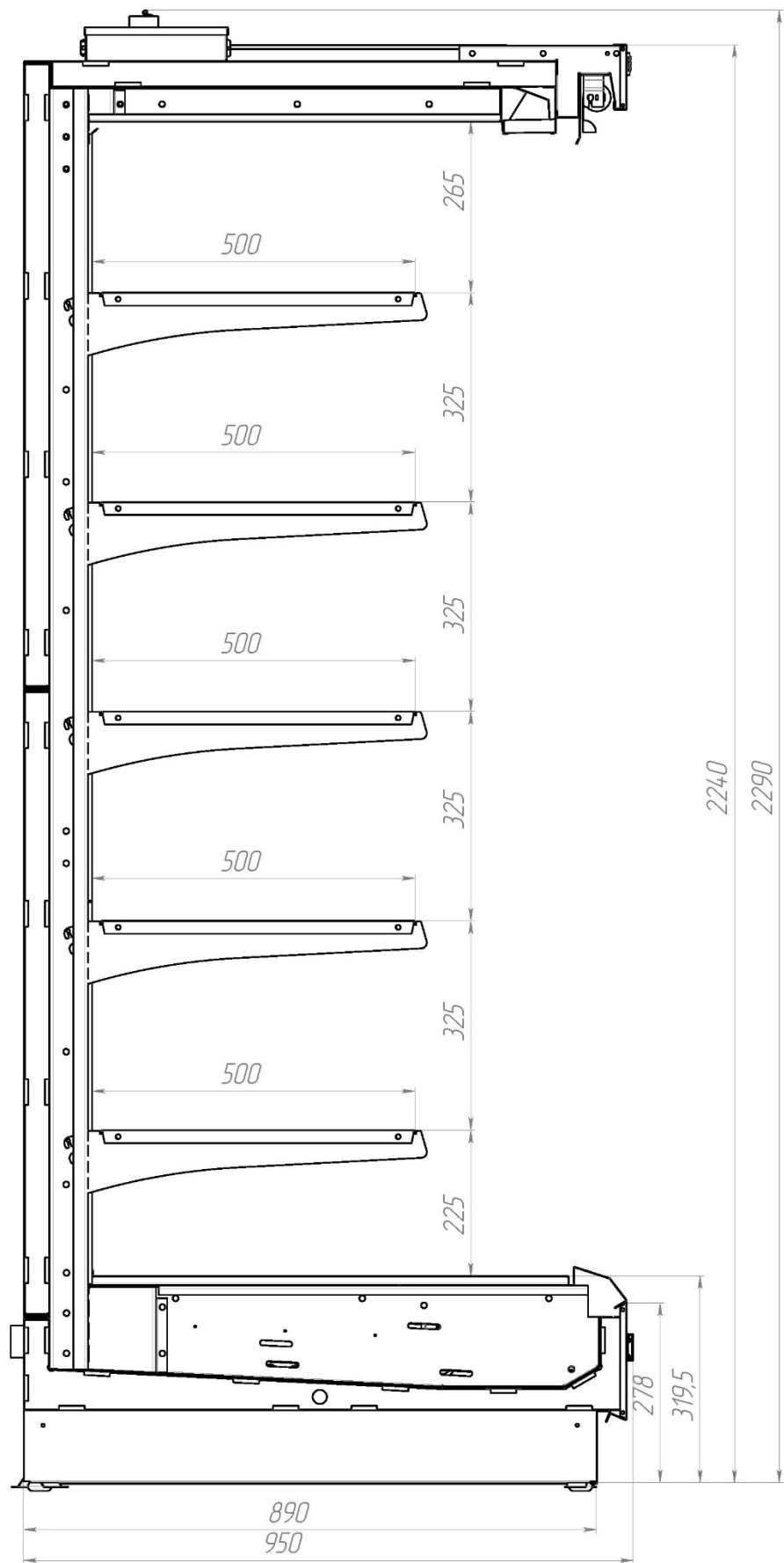
рисунк 2.6 – Сечение витрины VRIII2240.950
