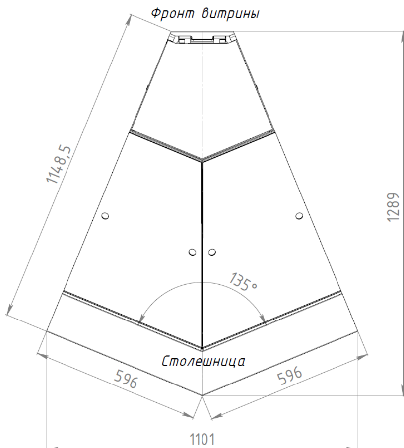
Витрина CALYPSO 3У 45 (вид сверху) рисунок 2
