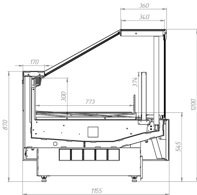
Витрина CALYPSO низкотемпературная
