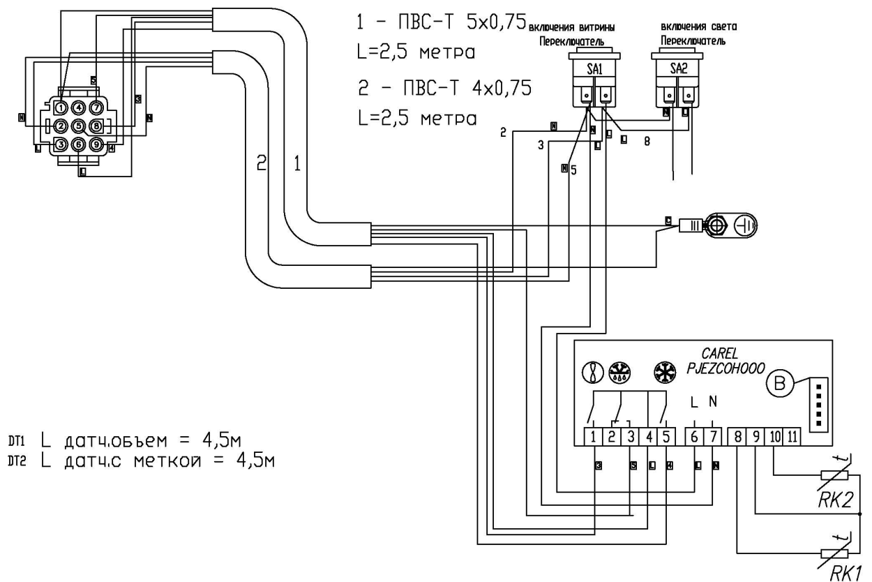
Схема электрическая монтажная кабельного шлейфа CRONOX PLUG-IN 375 PJEZCOH000
