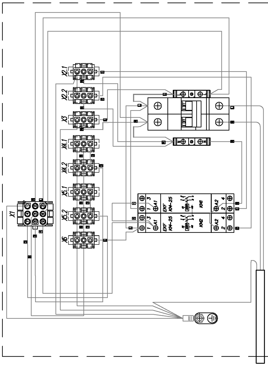
Приложение В Схема электрическая монтажная блока электросоединений CRONOX 250 / 375 (без реле времени)
