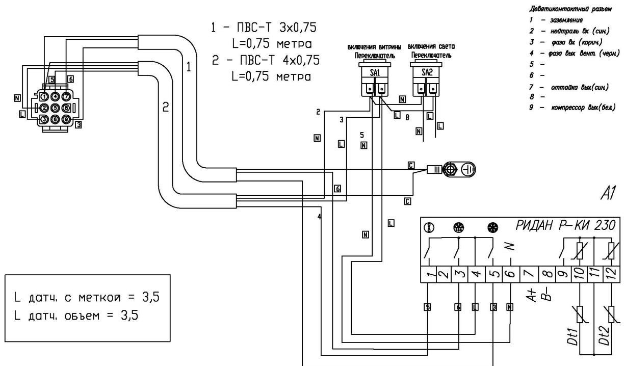
Схема электрическая монтажная кабельного шлейфа CRONOX plug in под РИДАН Р-КИ 230
