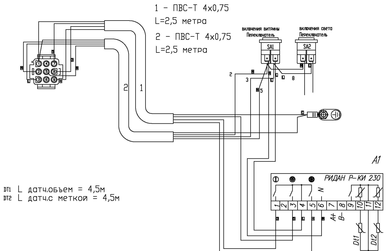
Схема электрическая монтажная кабельного шлейфа CRONOX PLUG-IN 375 РИДАН Р-КИ 230
