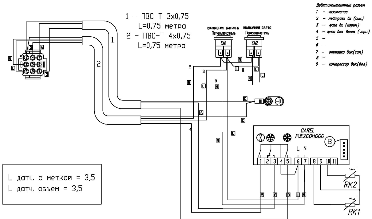
Схема электрическая монтажная кабельного шлейфа CRONOX plug in под CAREL PJEZCOH000
