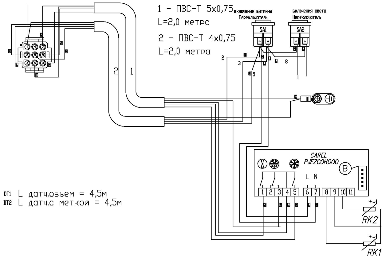
Схема электрическая монтажная кабельного шлейфа CRONOX PLUG-IN 250 PJEZCOH000
