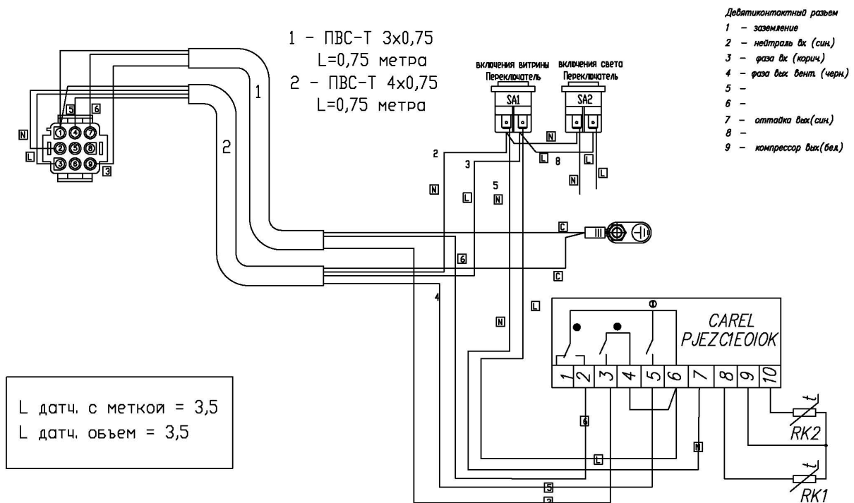
Схема электрическая монтажная кабельного шлейфа CRONOX plug in под CAREL PJEZC1EO1OK
