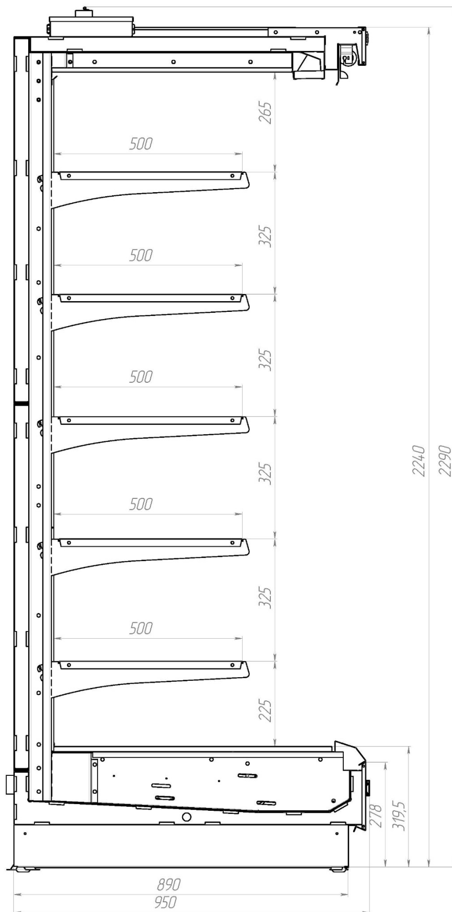
рисунк 2.6 – Сечение витрины VRIII2240.950
