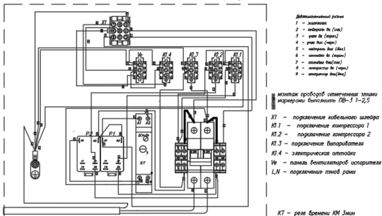
Приложение В Схема электрическая монтажная блока электросоединения TESEY II PLUG IN 125
