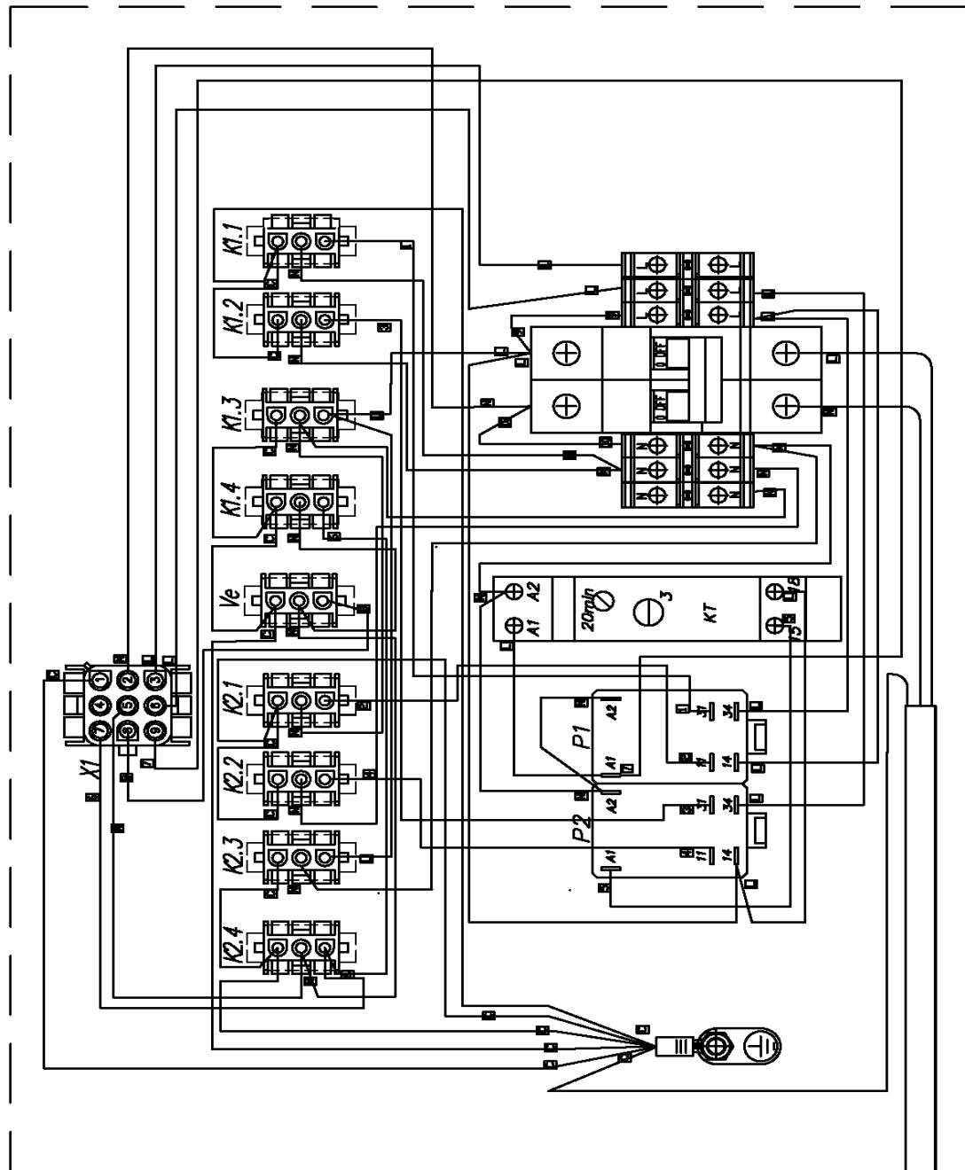
Схема электрическая монтажная блока электросоединений TESEY II PLUG IN 250
