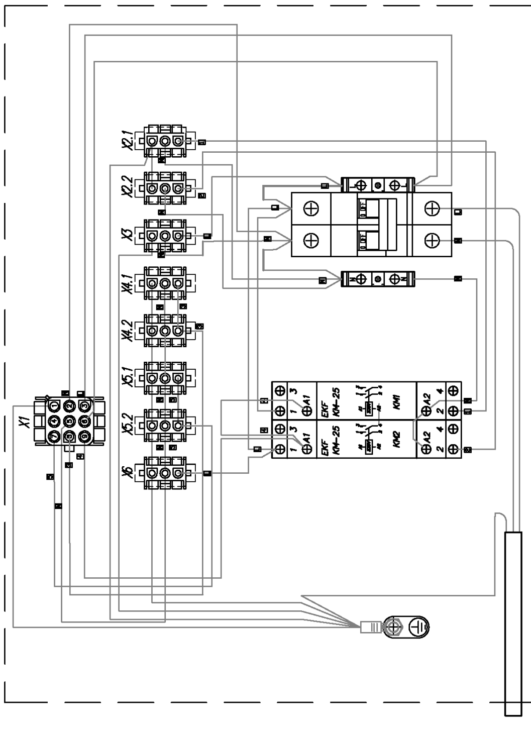
Приложение В Схема электрическая монтажная блока электросоединений CRONOX 250 / 375 (без реле времени)
