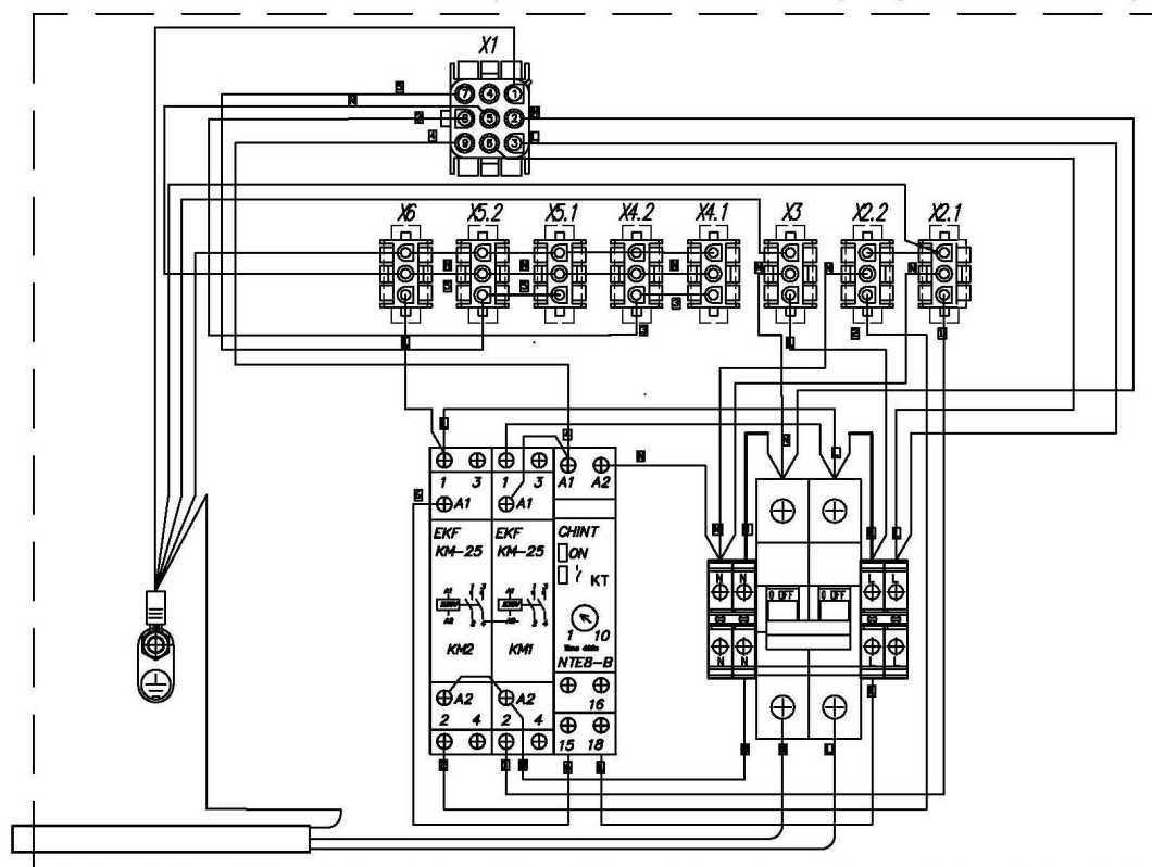
Приложение В Схема электрическая монтажная блока электросоединений CRONOX 250 / 375
