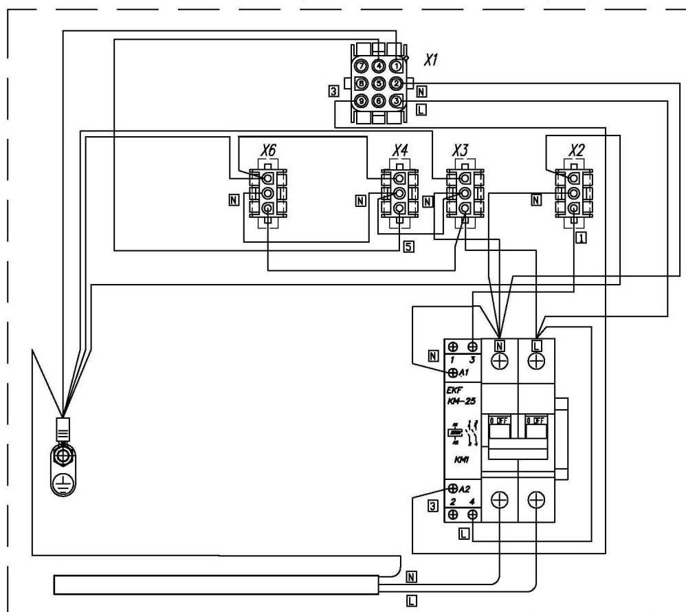
Приложение В Схема электрическая монтажная блока электросоединений CRONOX PLUG-IN 125/190
