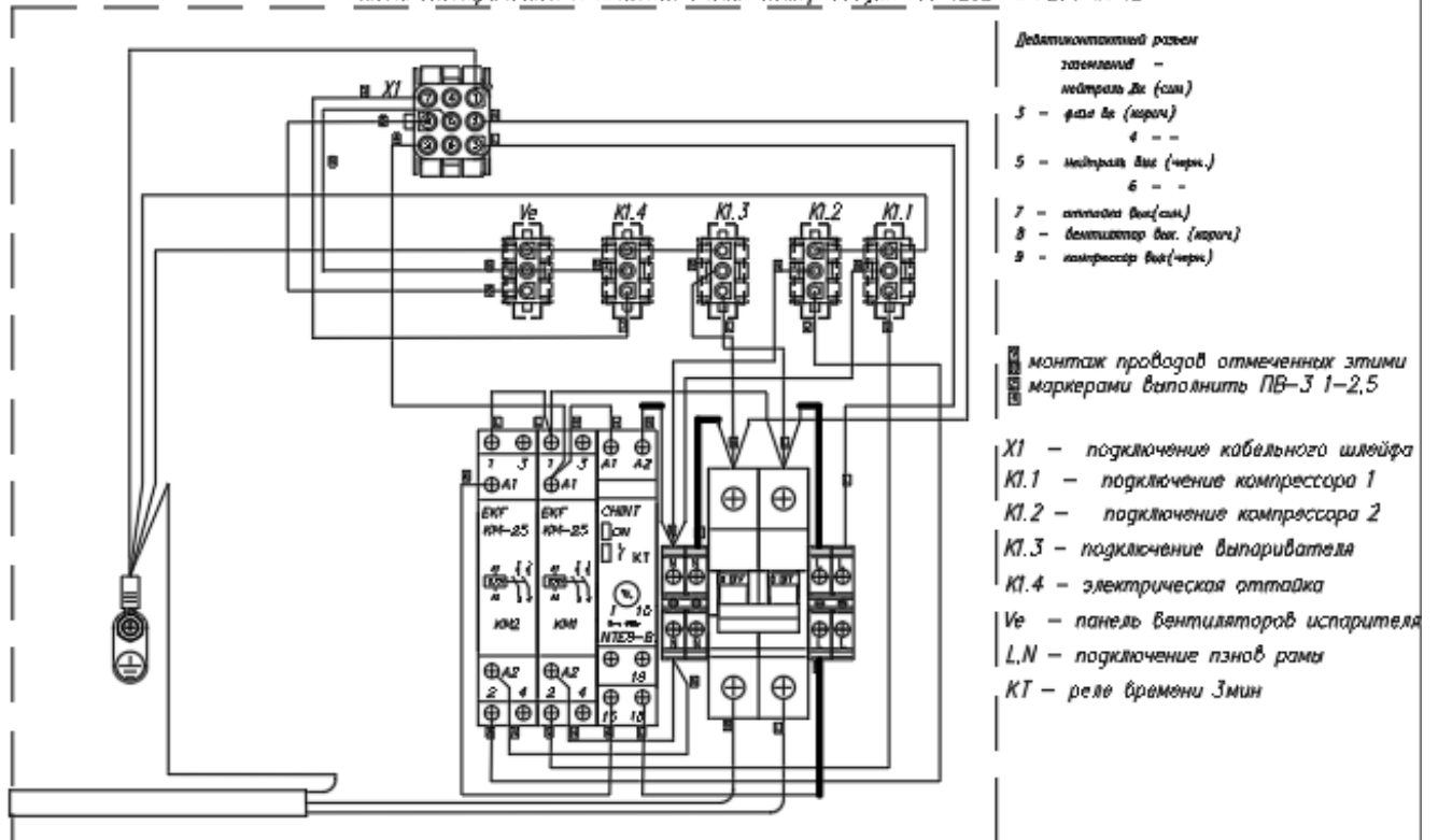
Схема электрическая монтажная блока электросоединения TESEY II PLUG IN 125
