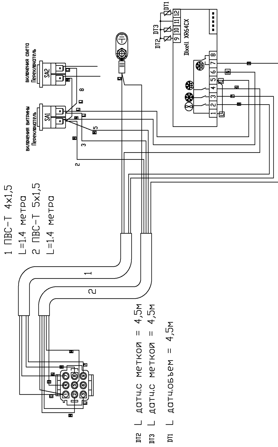
Схема электрическая монтажная шлейфа TESEY II PLUG IN 250
