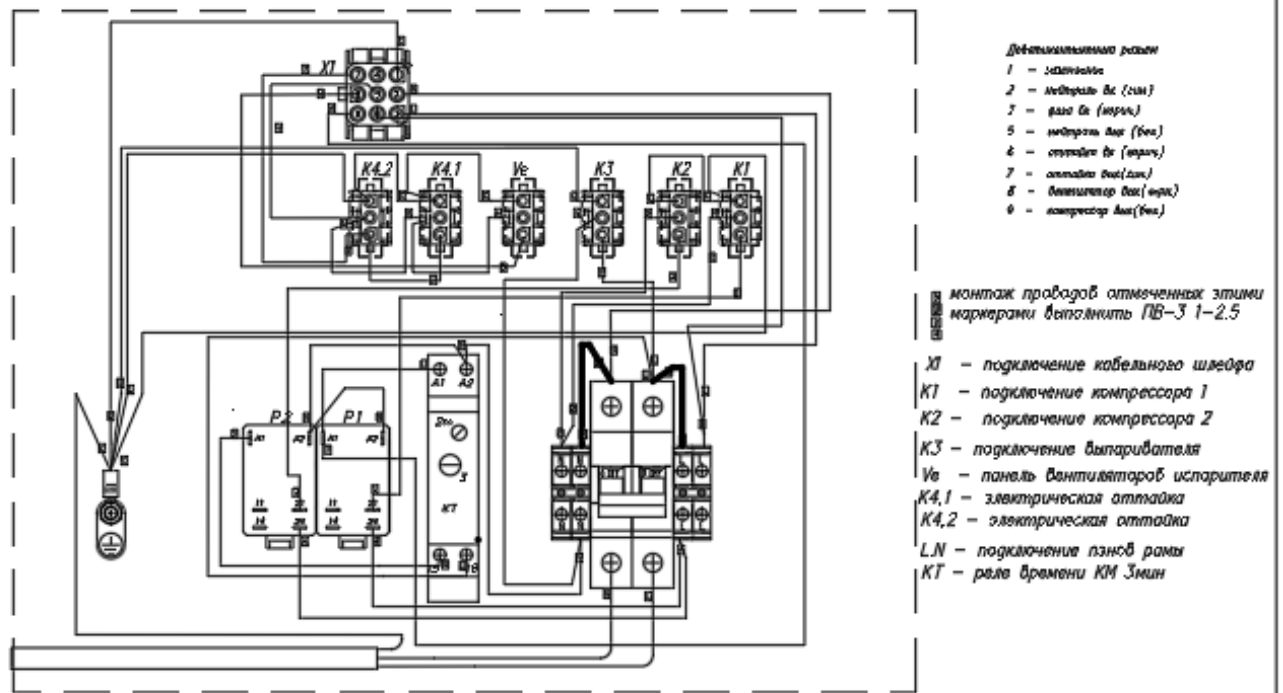
Приложение В Схема электрической монтажной блока электросоединений TESEY II PLUG IN 190
